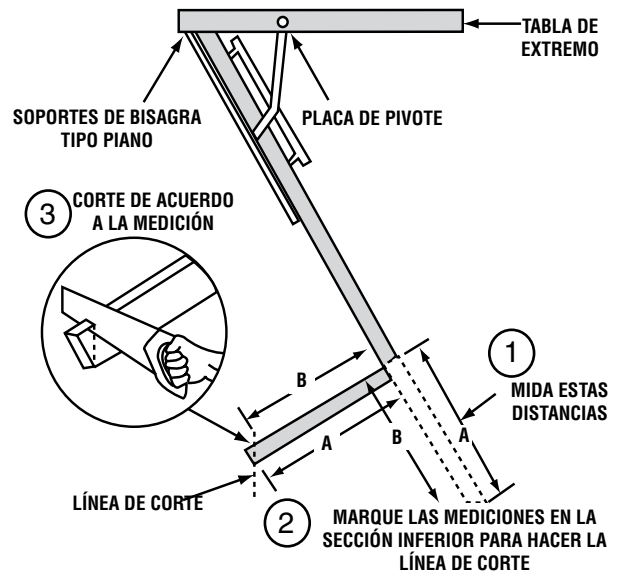
FIGURA 4A - AJUSTE SEGÚN LA ALTURA DEL CIELO RASO
