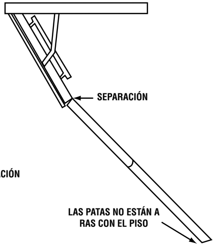
FIGURA 5B - INSTALACIÓN INCORRECTA
