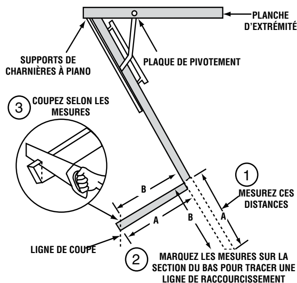
FIGURA 4A - AJUSTEMENT AUX HAUTEURS DE PLAFONDS
