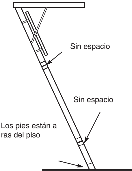
Disposición correcta
